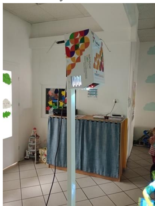
Rysunek 6. Statyw do mobilnej edukacyjnej podłogi interaktywno-multimedialnej
